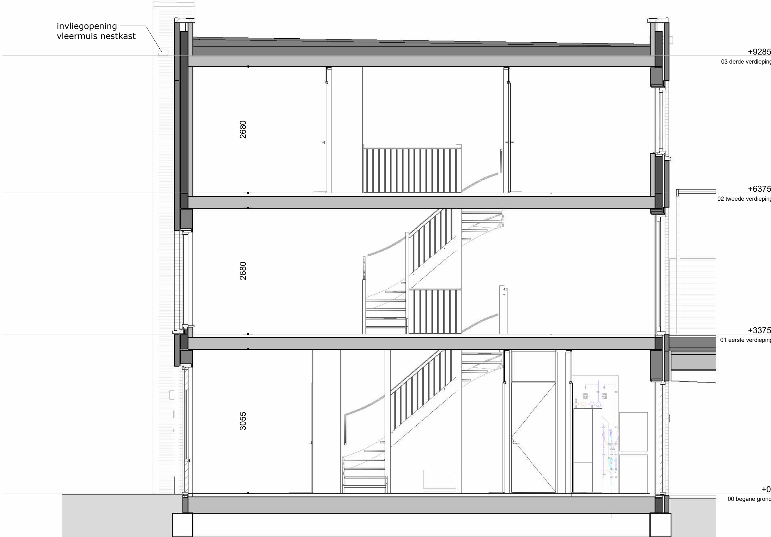
DOORSNEDE
