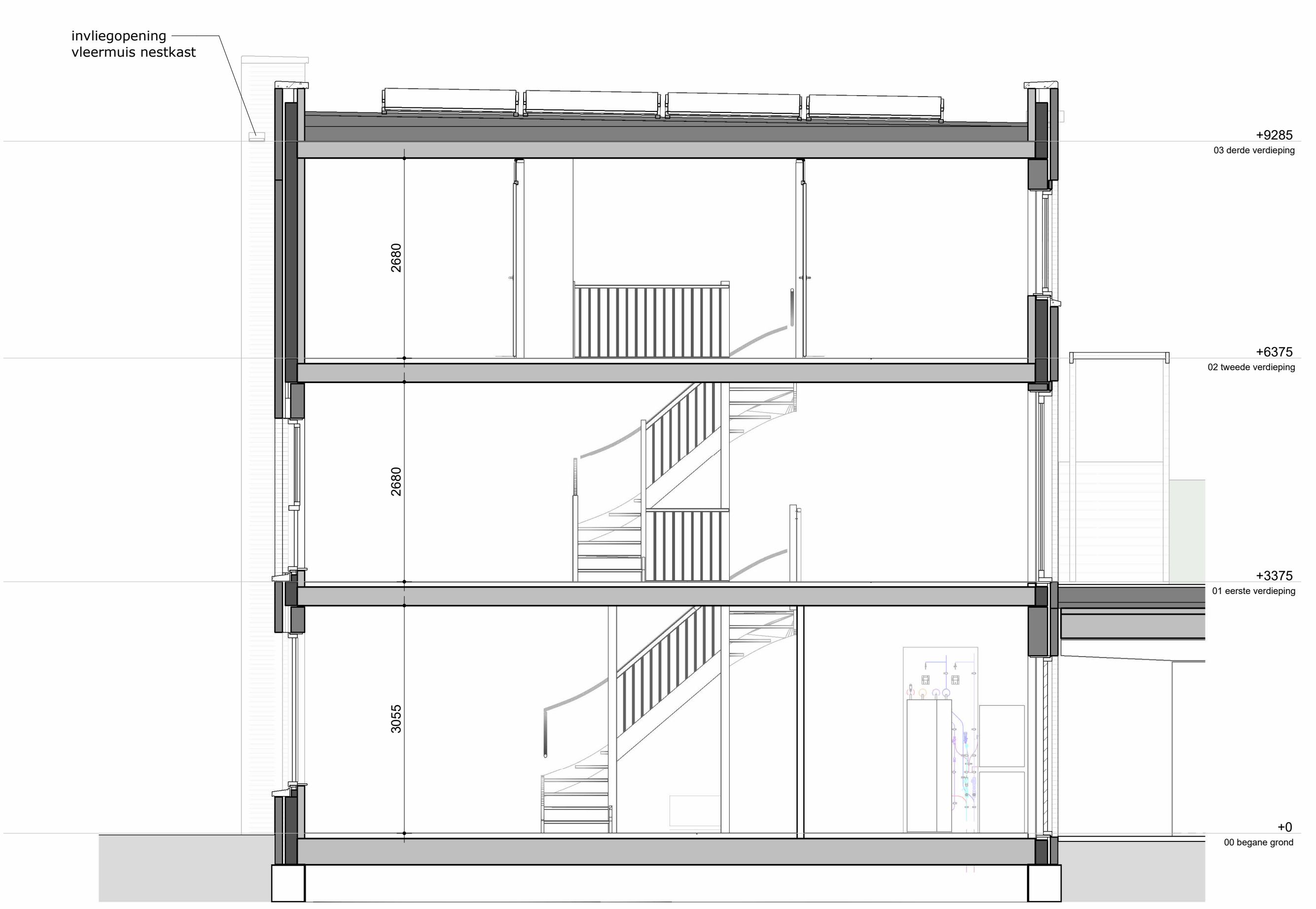
DOORSNEDE
