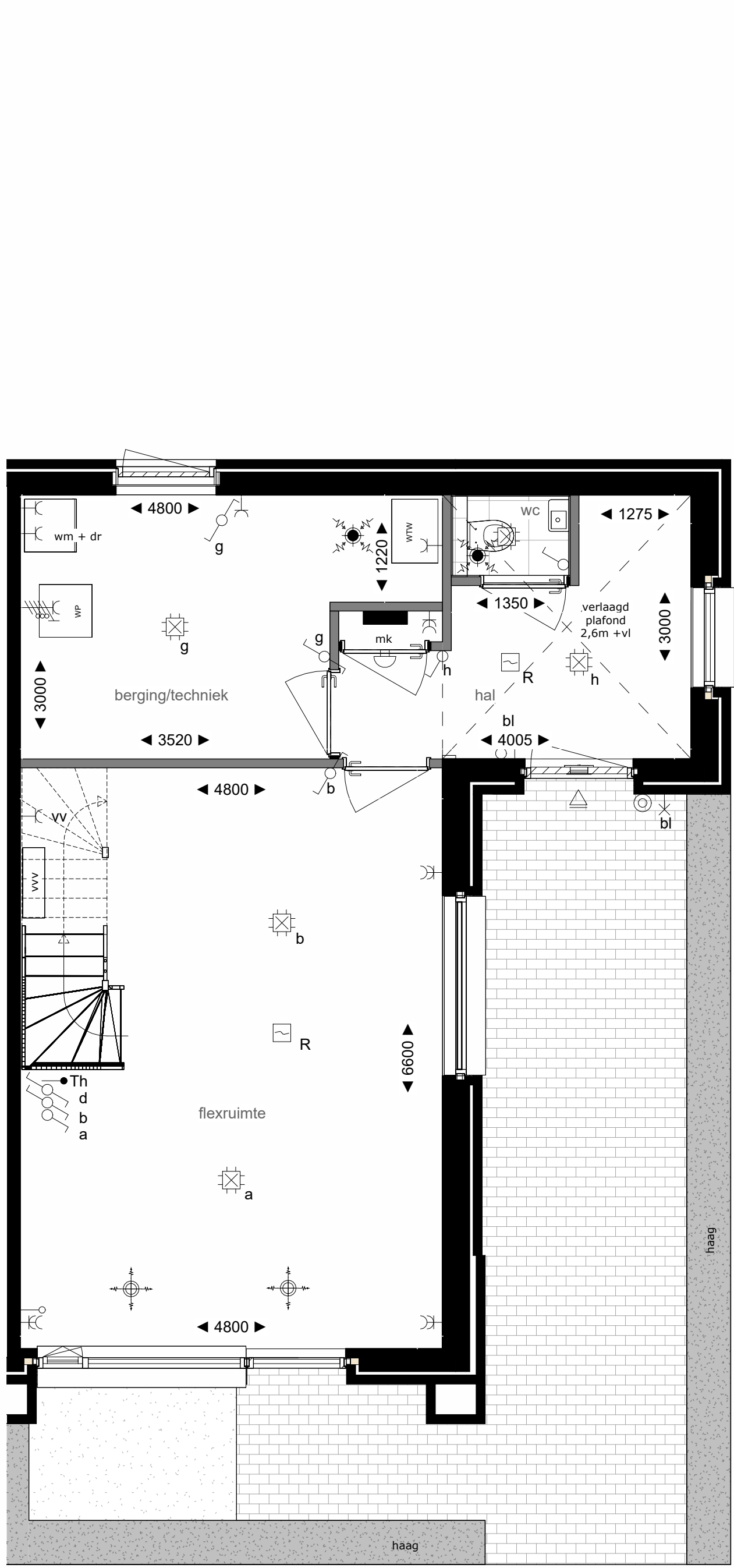
BEGANE GROND
