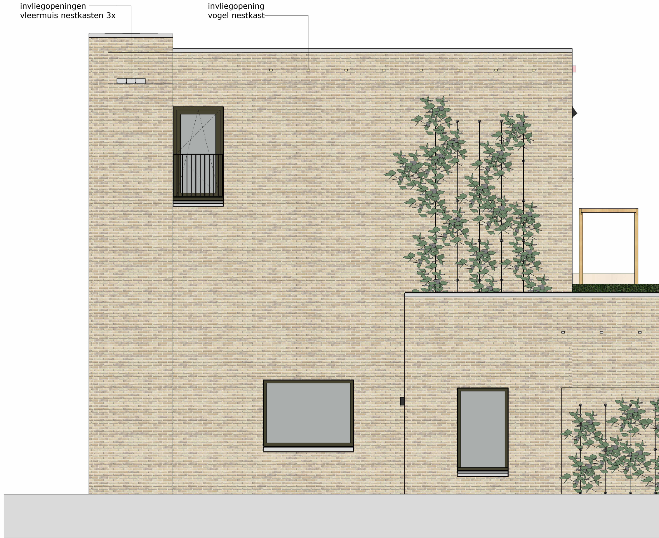
LINKERZIJGEVEL (noord)
