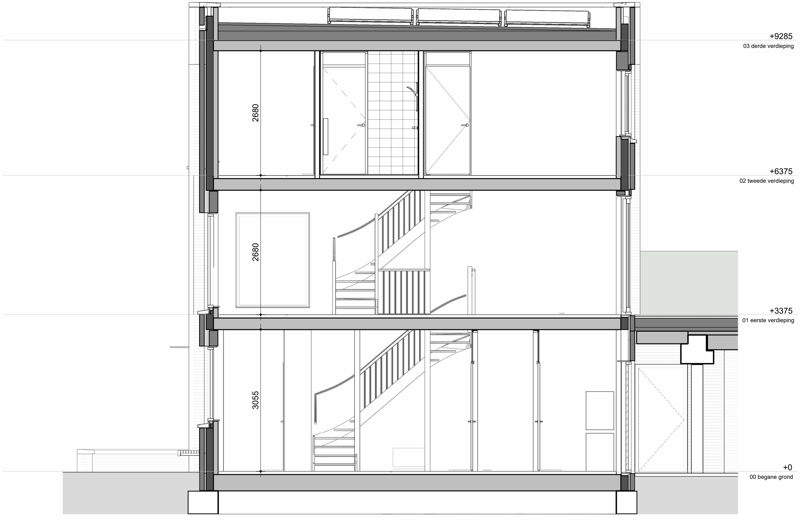
DOORSNEDE
