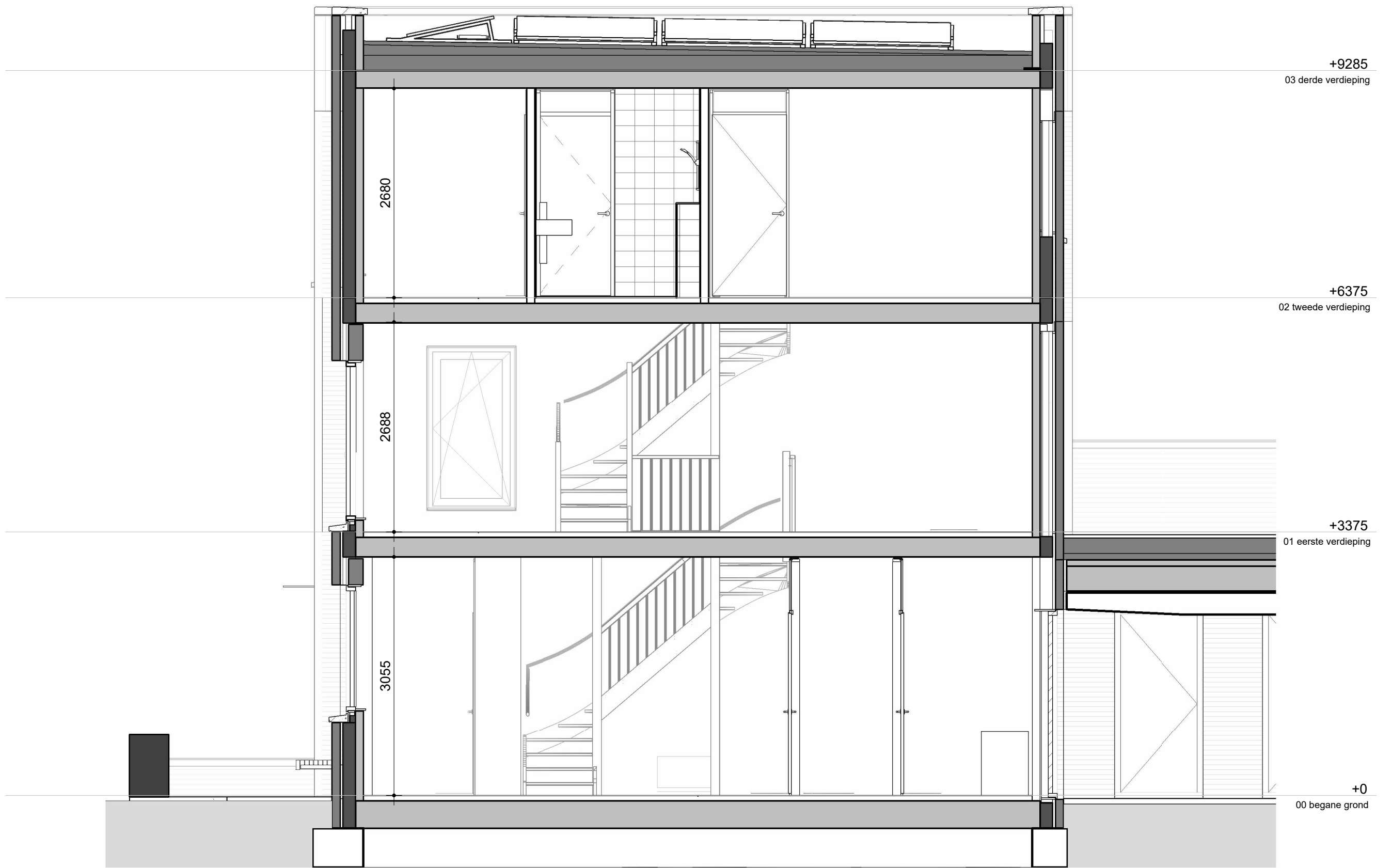
DOORSNEDE
