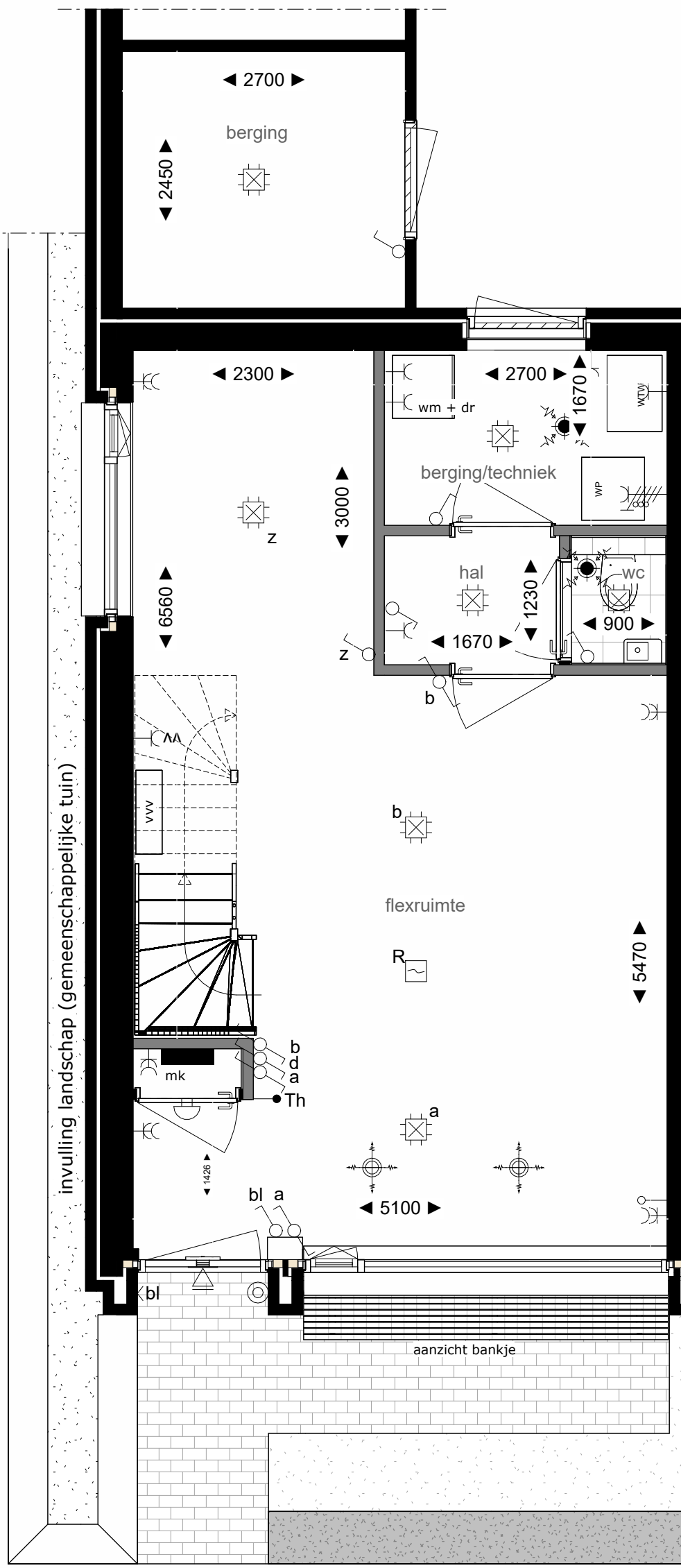
BEGANE GROND
