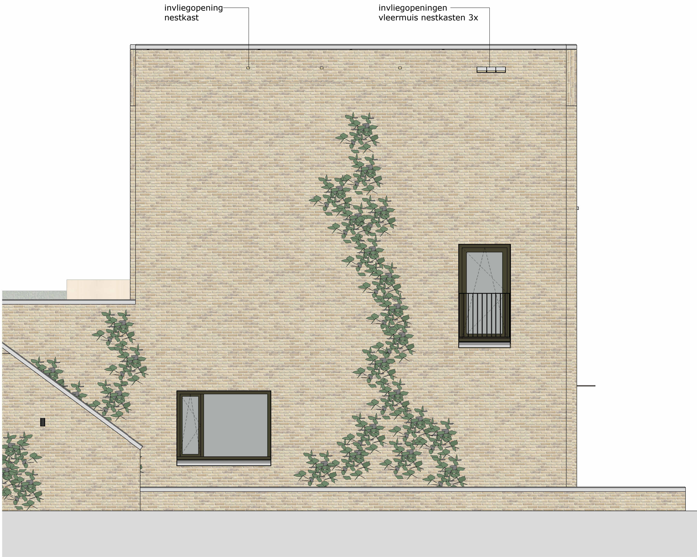
LINKERZIJGEVEL (noord)
