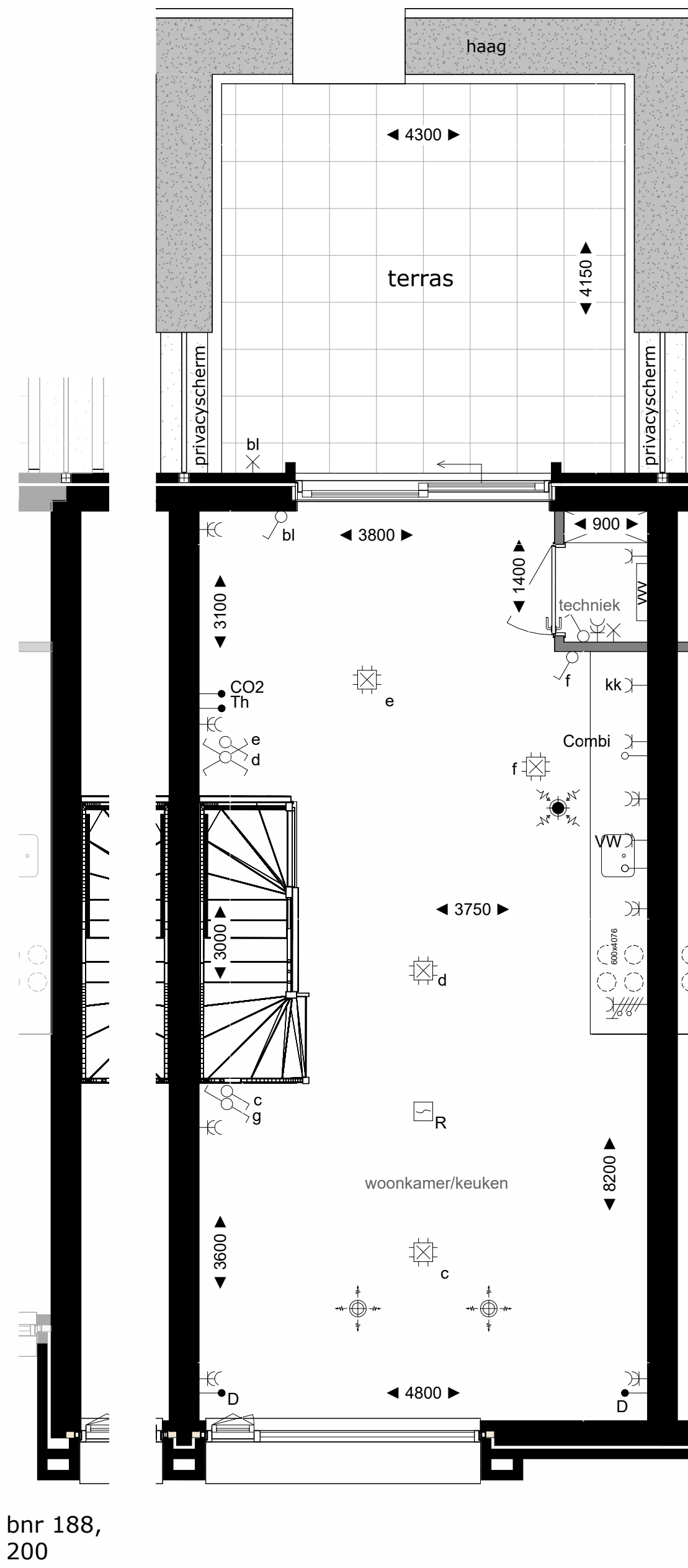
1e VERDIEPING
