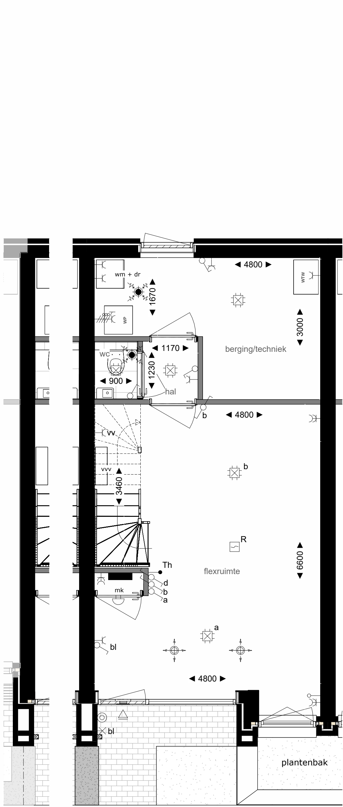
BEGANE GROND
