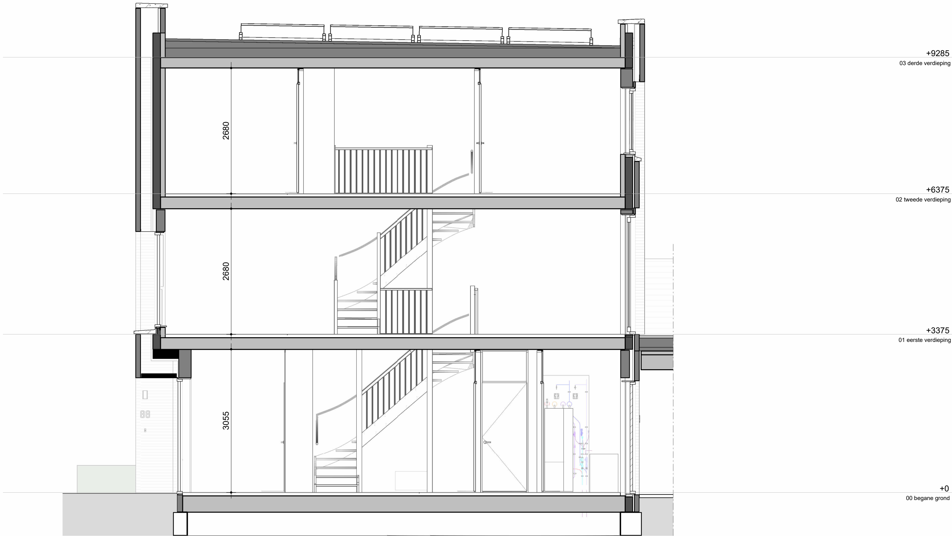
DOORSNEDE
