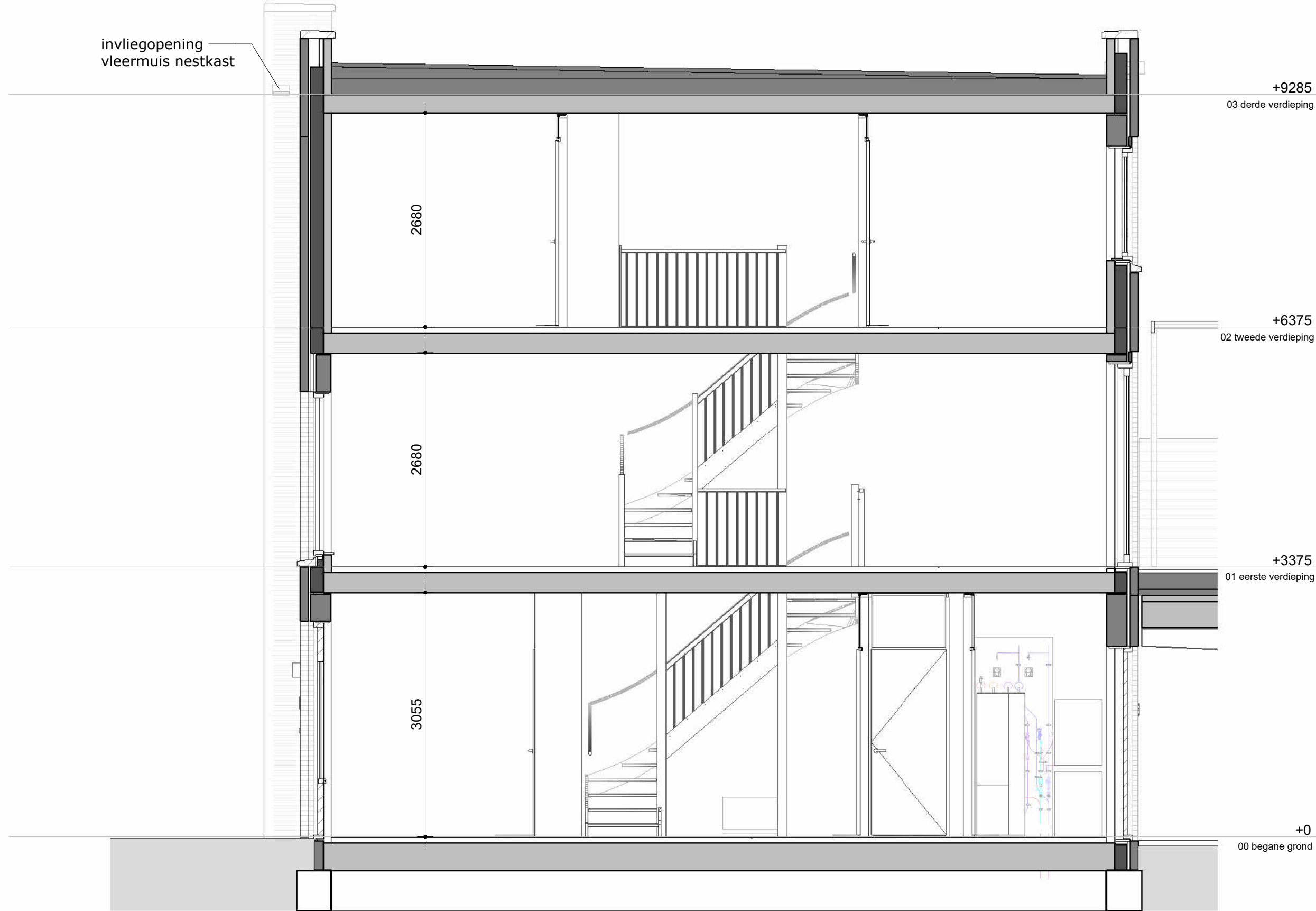
DOORSNEDE
