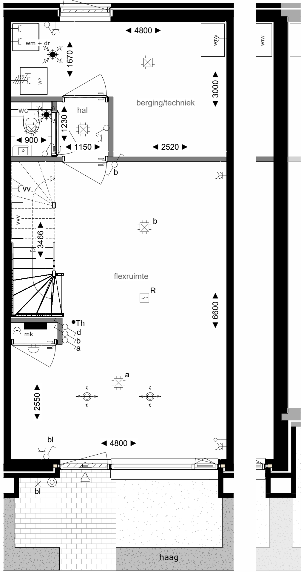
BEGANE GROND
