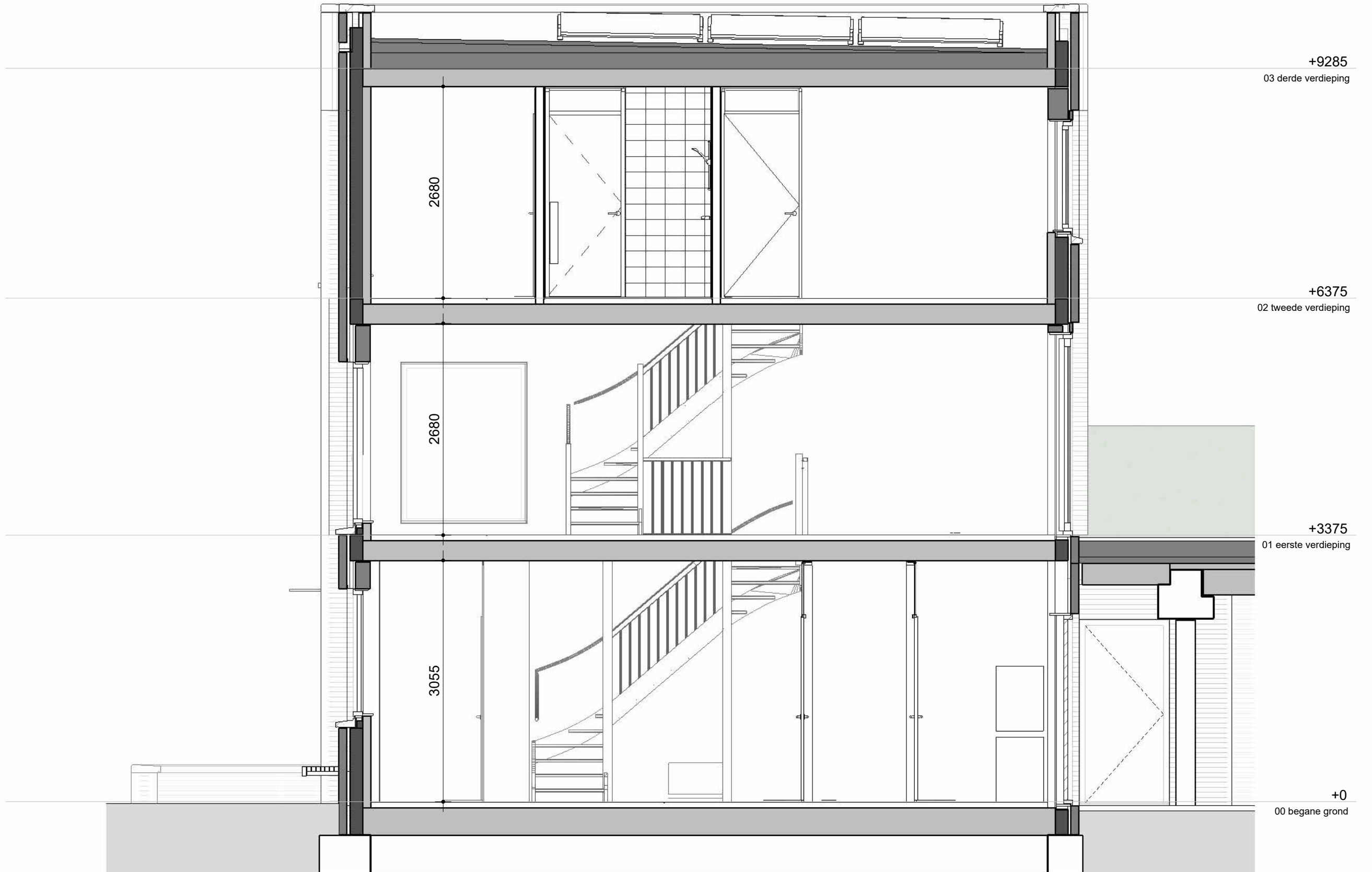
DOORSNEDE
