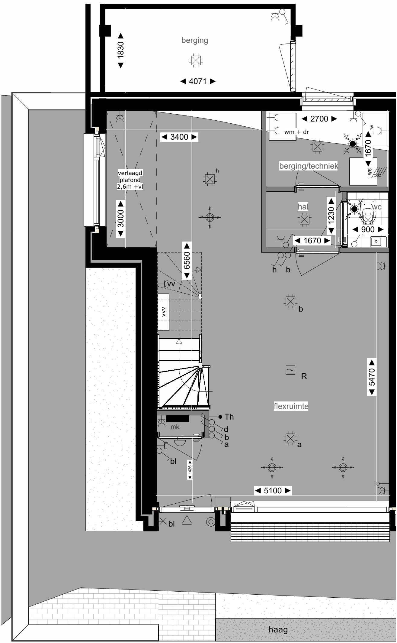
BEGANE GROND
