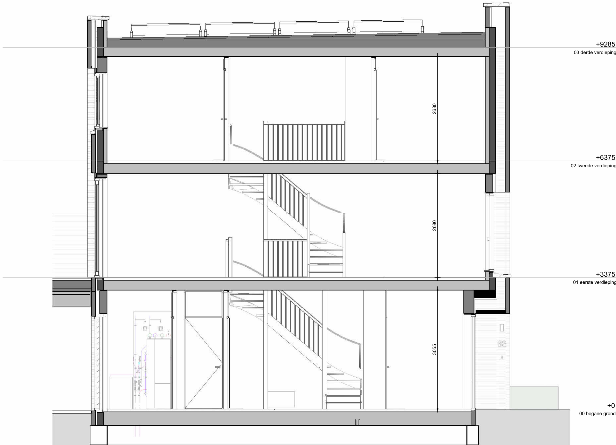
DOORSNEDE
