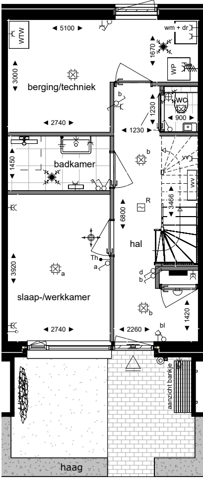
begane grond
