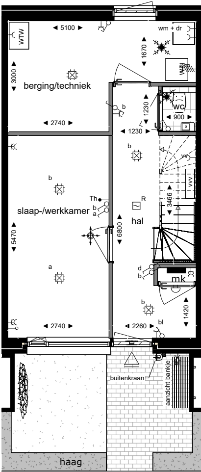
begane grond
