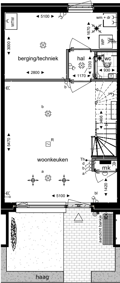
begane grond
