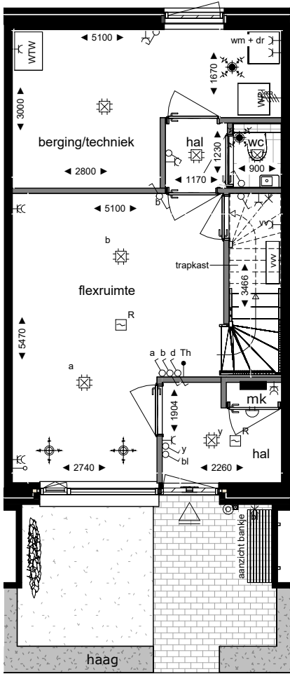
begane grond
