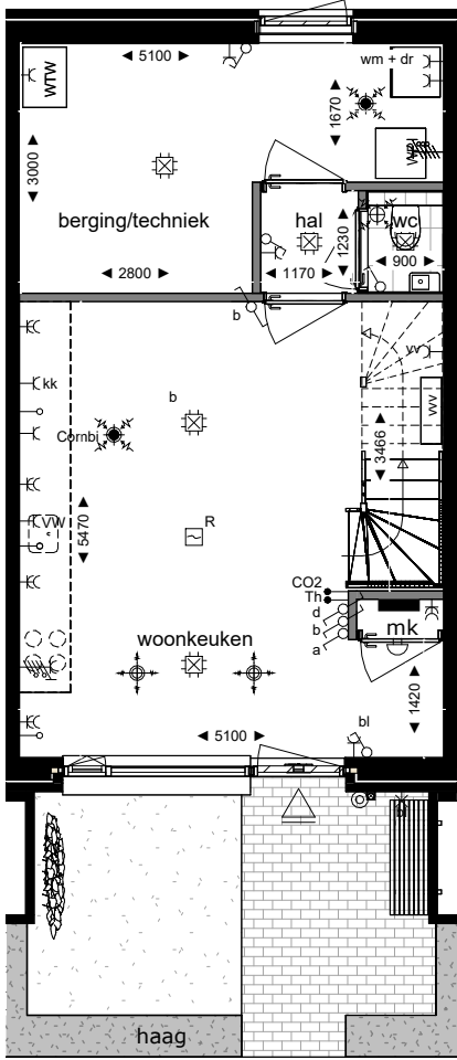
begane grond
